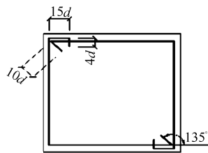
图4 开口箍示意
