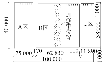
图1 平面布置示意
